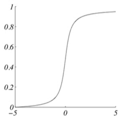
Fonction de répartition
