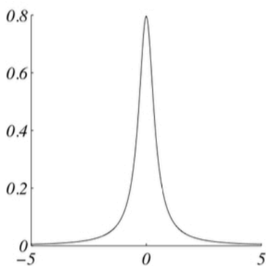
Densité de probabilité
