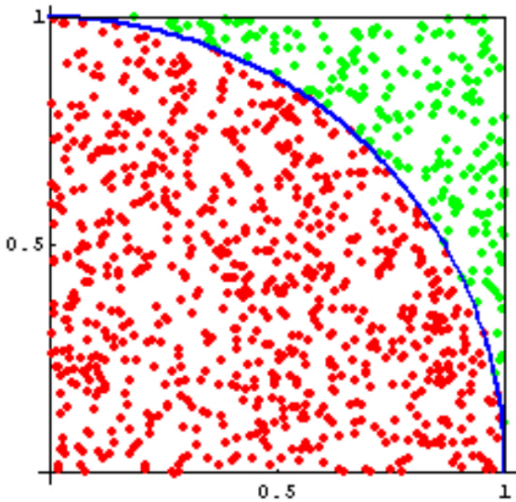
Approximation de \pi avec la méthode de Monte Carlo
